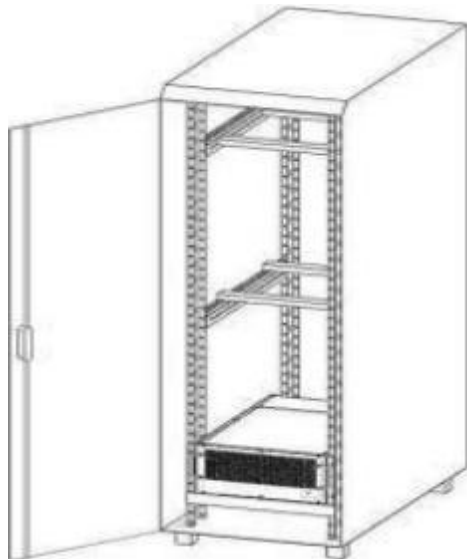
图 2.4 .2 为室内机安装位置示意图
