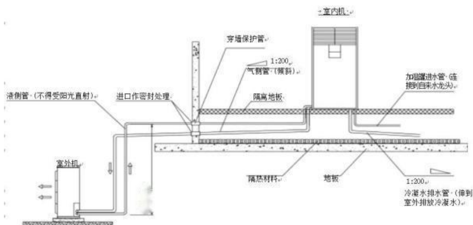
图 2.3.3 室内机高于室外机的安装示意图
